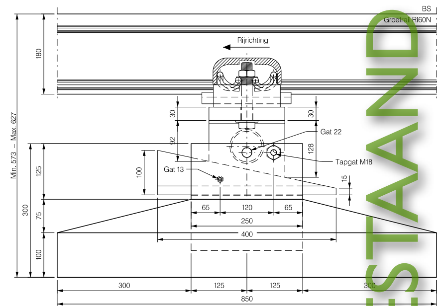
AANZICHT B-B
