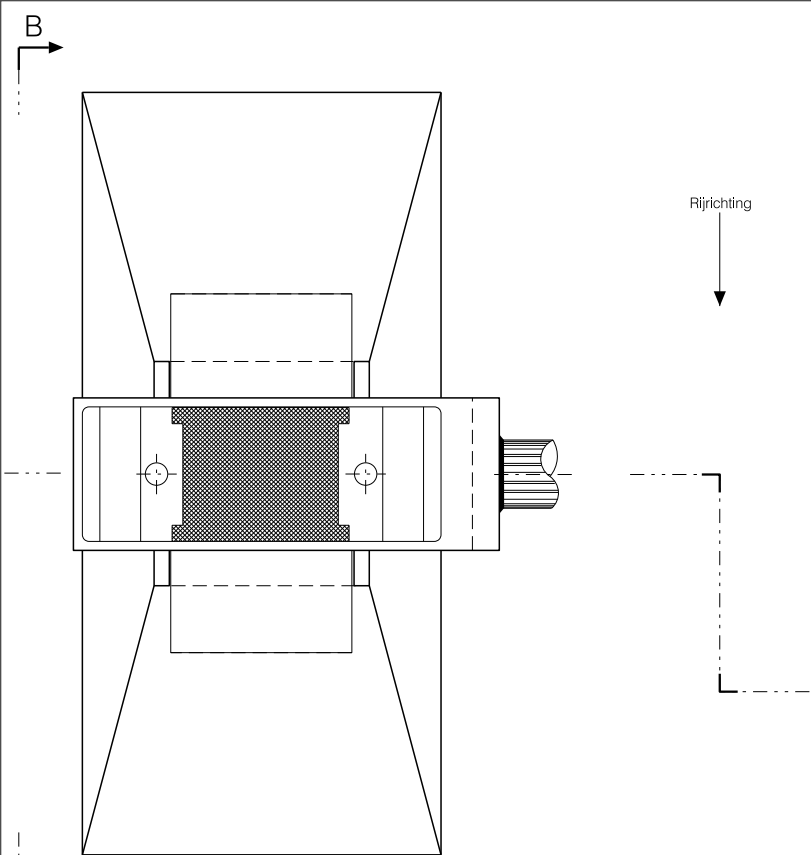
BOVENAANZICHT
